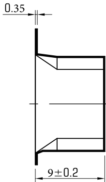
A-A剖面
