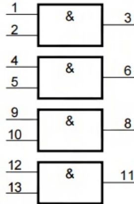
图 2 IEC 逻辑符号
