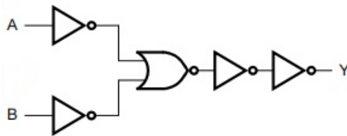
图 3 逻辑框图
