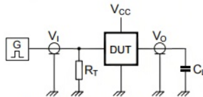
图4 测量开关时间的测试电路
