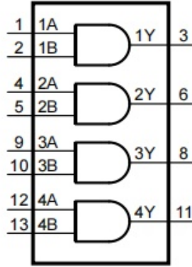
图 1 逻辑符号
