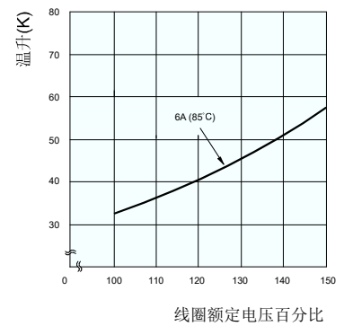
线圈温升
