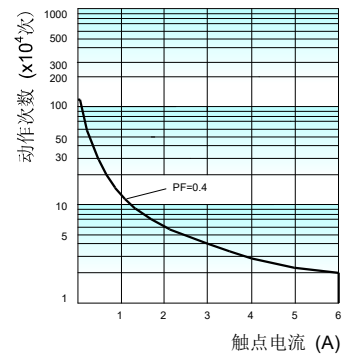
交流感性负载电耐久性曲线
