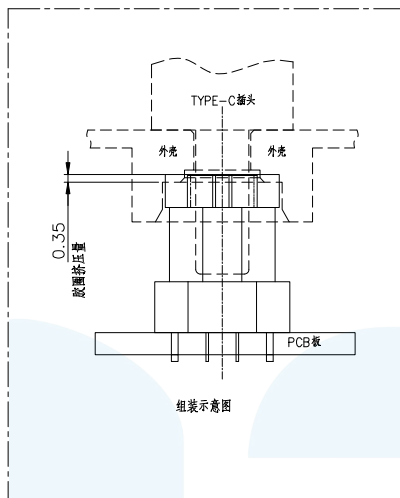
组装示意图
