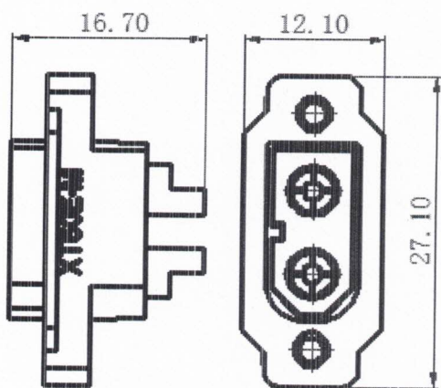
XT60E-M
