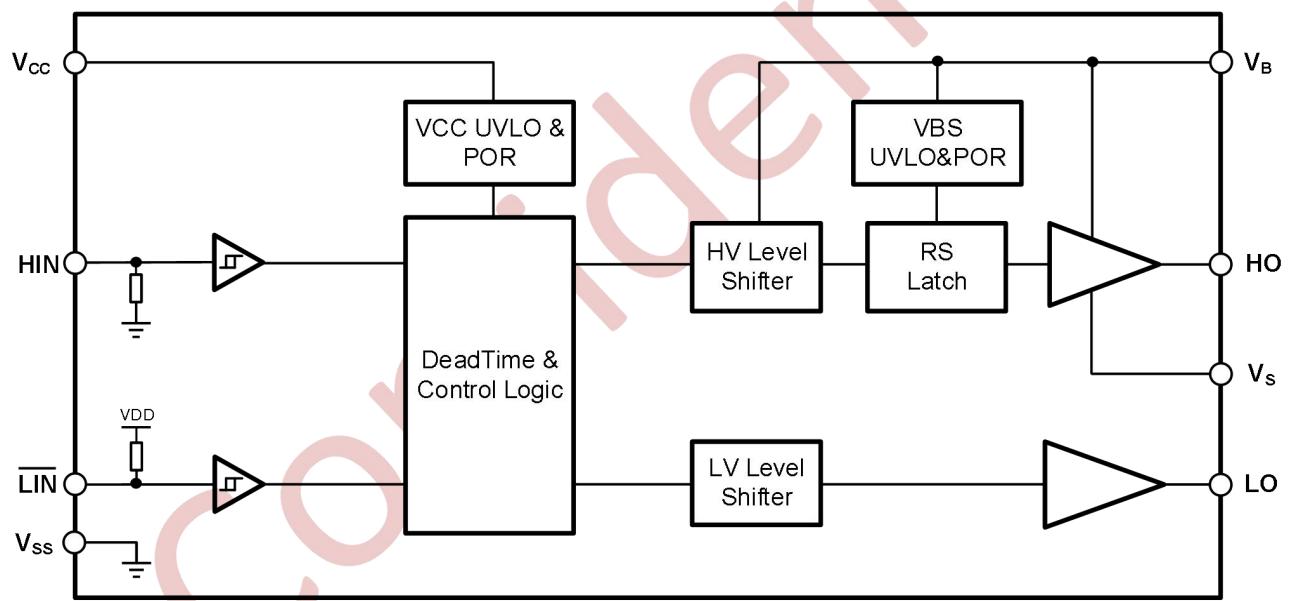
图 10-1 XJNG2103C 功能框图
