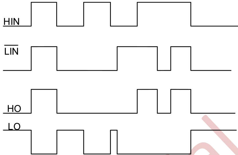
图 9-1 XJNG2103C 输入输出时序波形
