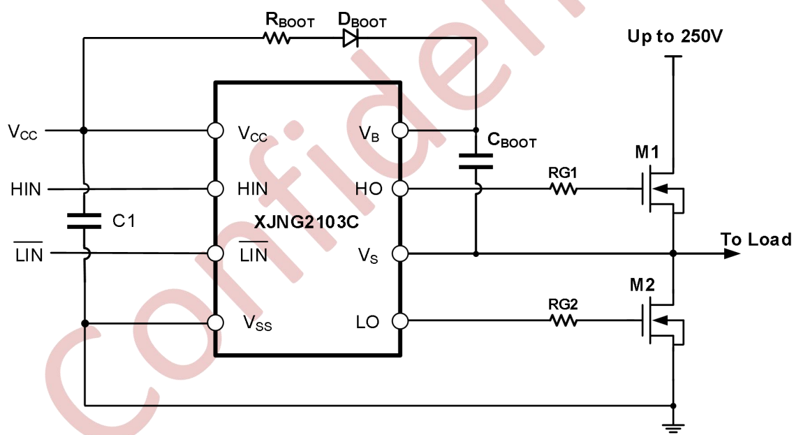
图 11-1 典型应用电路图
