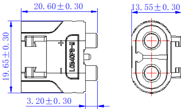
互配尺寸 Matching size
