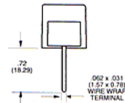
6 - Wire Wrap Pin
