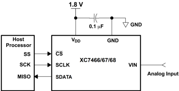
电路连接图
