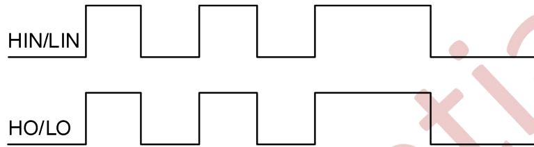
图 9-1. NSG2106 输入输出时序波形
