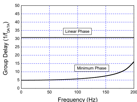
Fig. 26 FIR Group Delay ( f_{DATA} = 500\text{Hz} )
