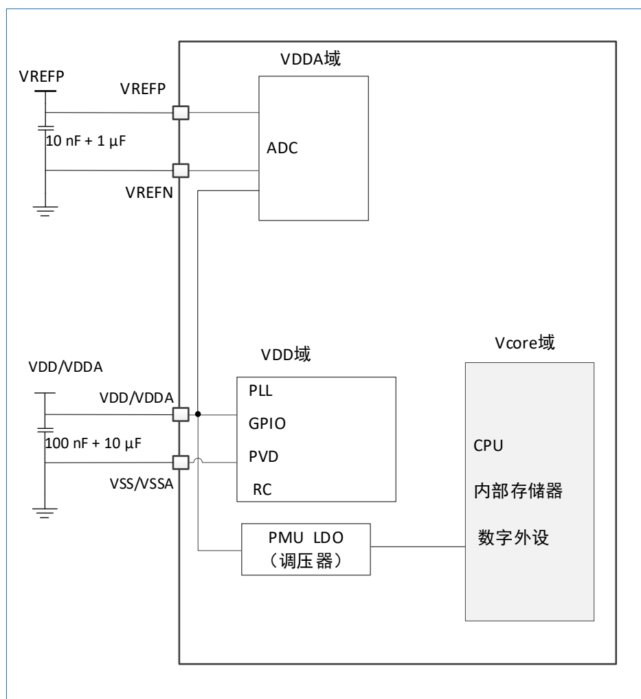
图 5-1 电源框图
