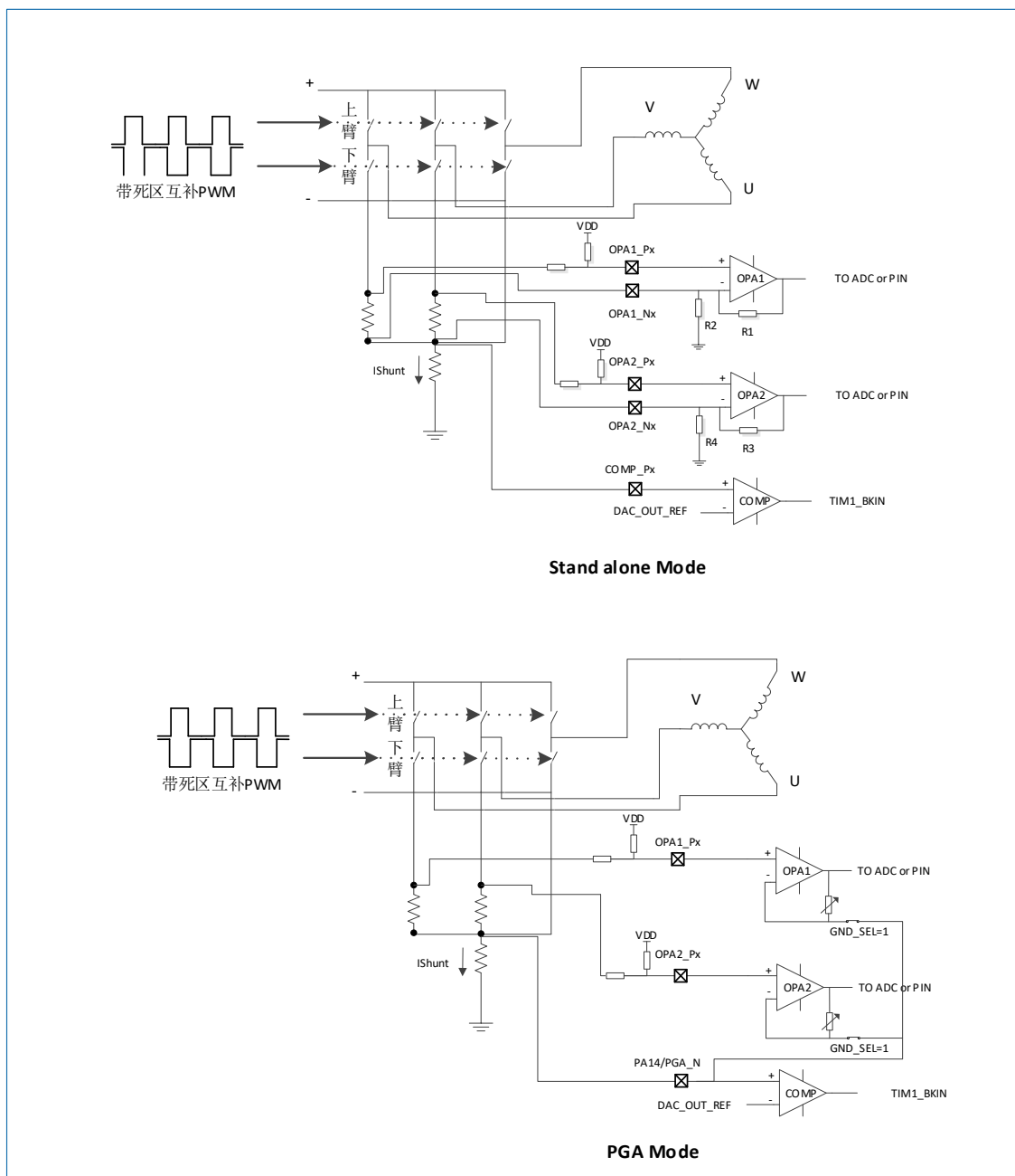
图 5-2 运放应用
