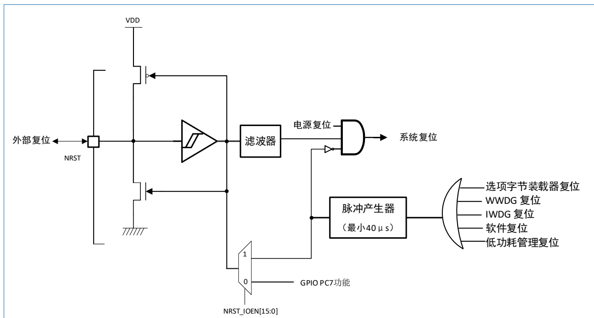
图 3-3 复位信号
