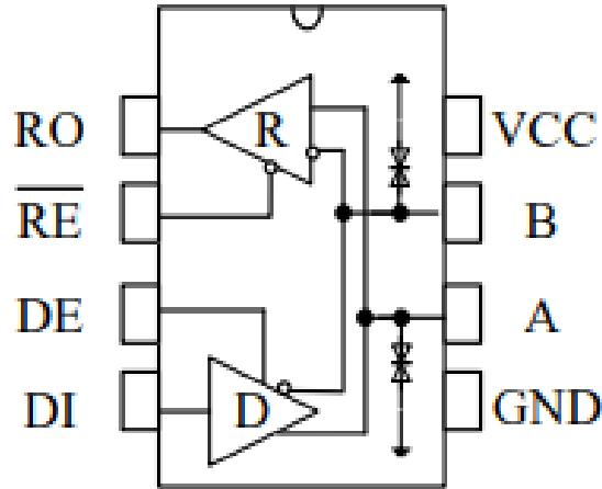
图 1 MAX3485EESA+T 引脚分布图
