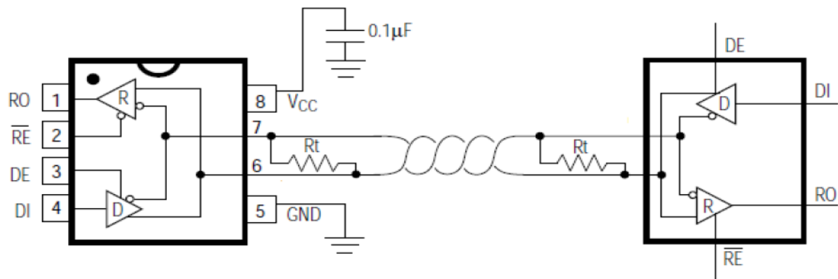
图 1: MAX483ECSA-TD典型半双工应用电路
