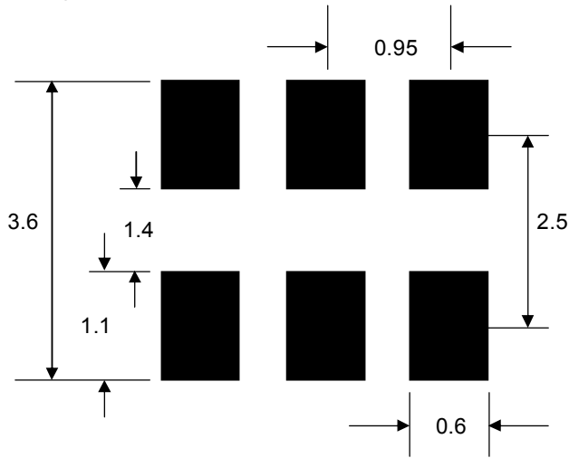
Package : SOT23-6L
