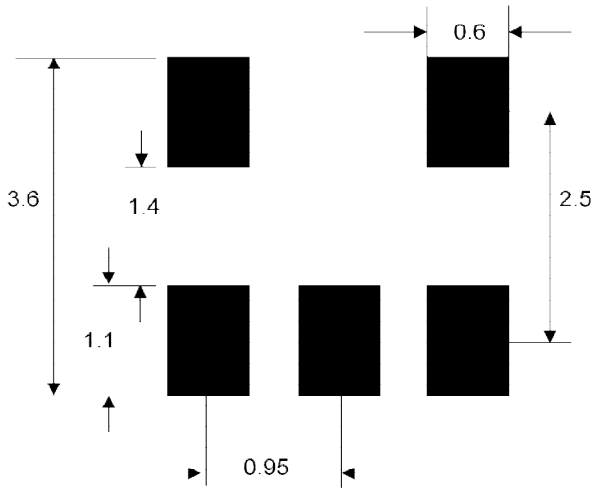
Package : SOT23-5L
