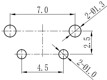
PCB线路板安装图(±0.1)
