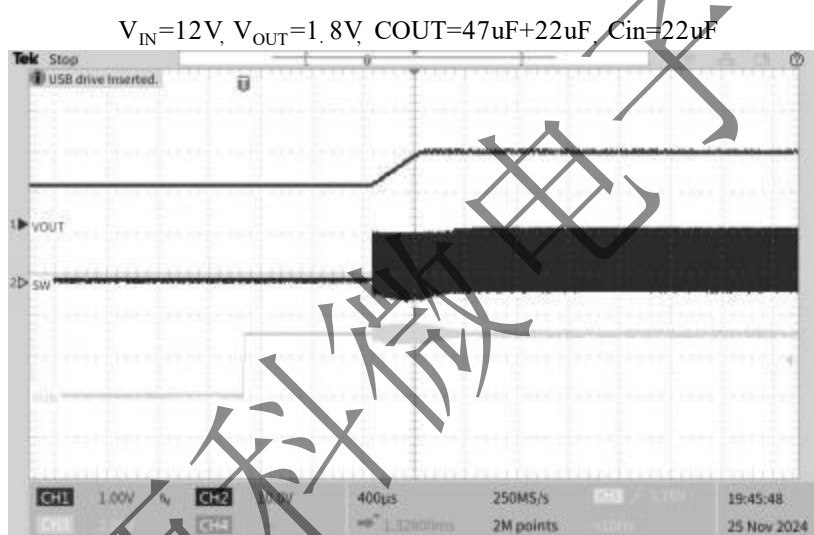
图 17 启动预偏置输出
