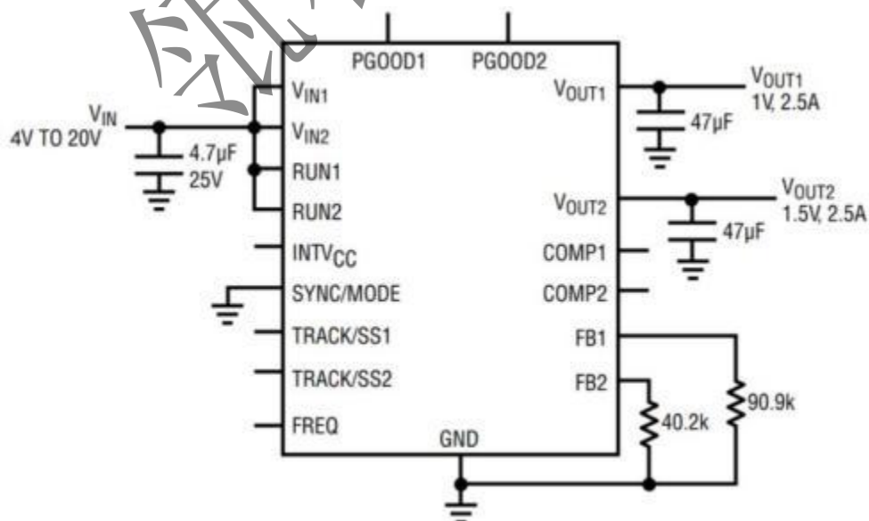
图 1 典型应用图
