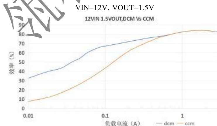
图 3 突发模式效率 VS 连续模式效率
