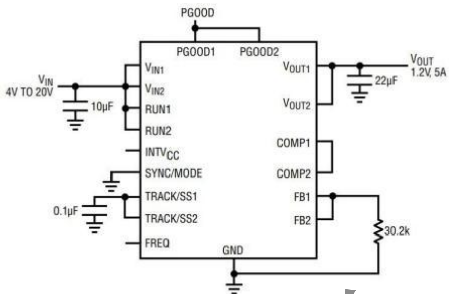
图 22 并联 6A 设计中的 4V_{IN} \sim 20V_{IN} \sqrt{1.2V} 两相
