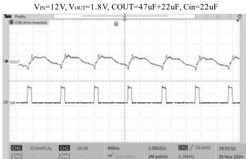
图 16 输出纹波
