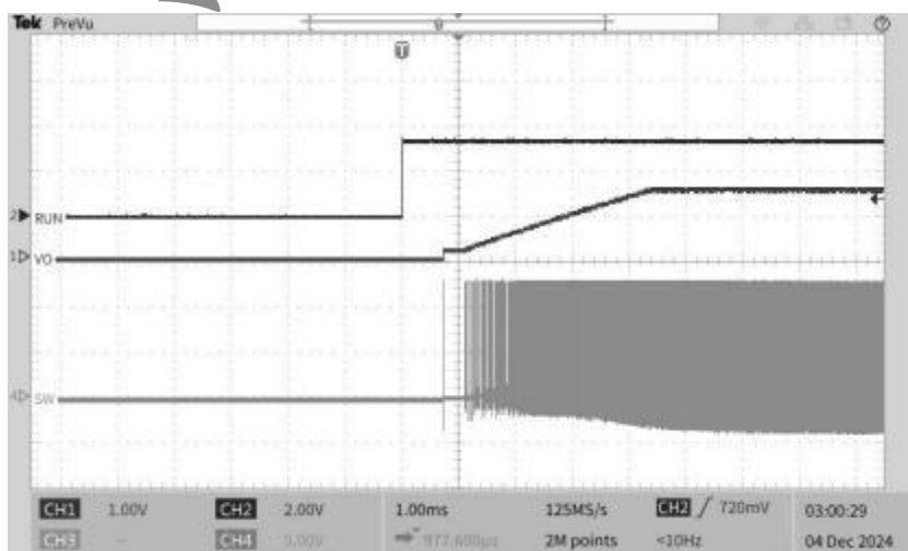
图 12 带载 2.5A 启动
