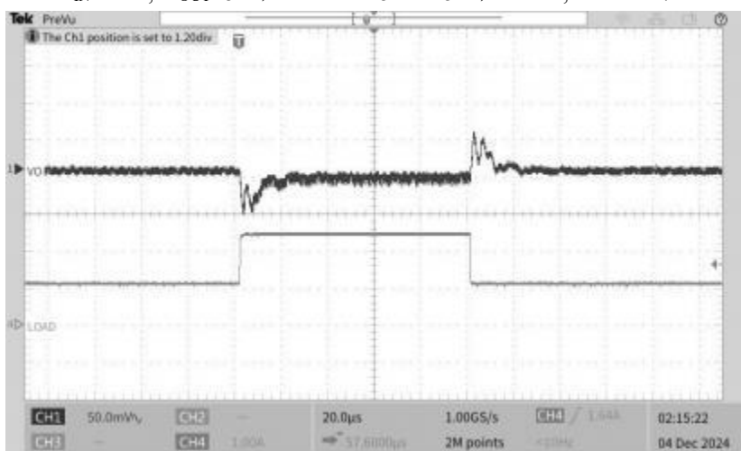
图 10 输出瞬态响应, V_{OUT}=5V
