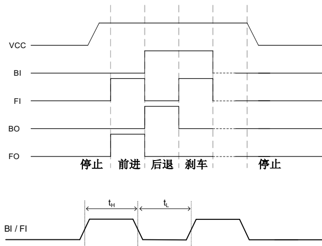
图 5. 输出时序图
