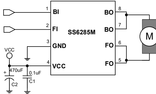
图 4. 应用原理图
