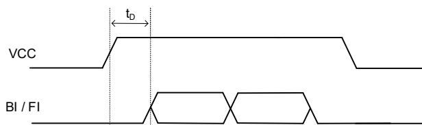
图 6. 上电时序图
