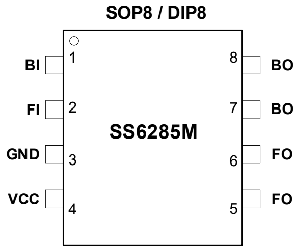
图 1. 顶视图
