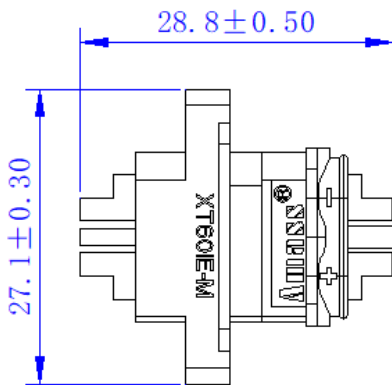
互配尺寸 Matching size
