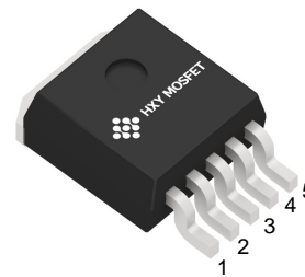
TO-263-5L (TO-263-5)
