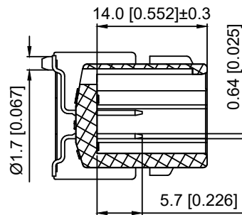
SEC:A-A
