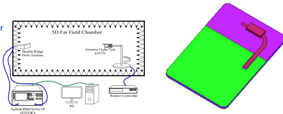
Fig.2 暗室示意图
