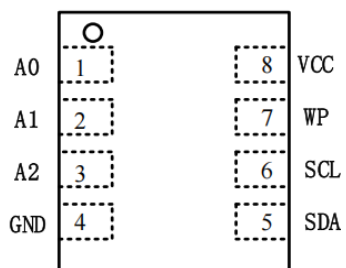
8 -pad DFN
