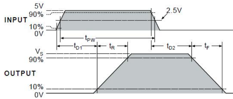
图 9-1 输入输出(同相)波形图
