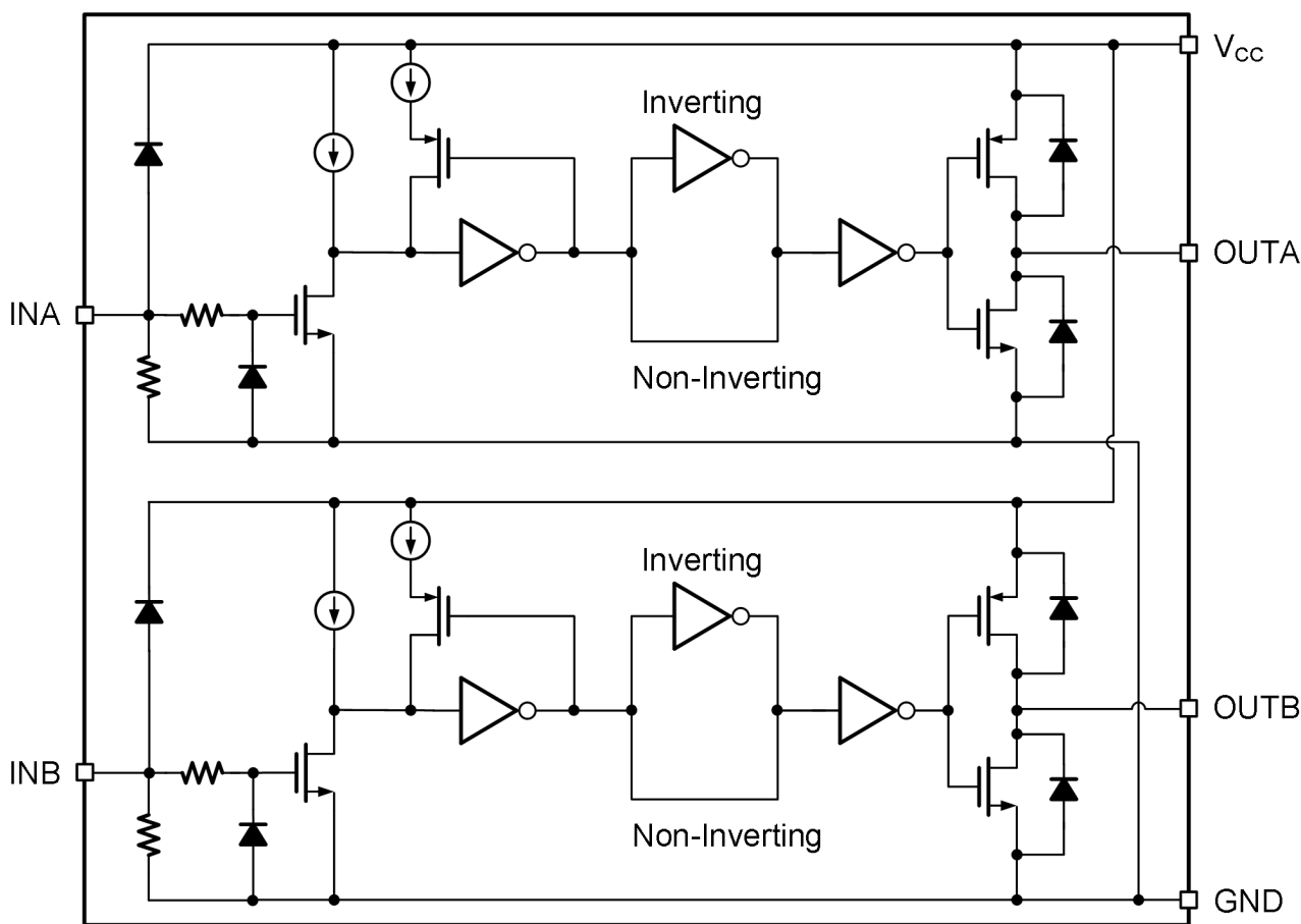
图 10-1 NSG4427 功能框图
