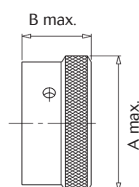
Receptacle cap Type 9
