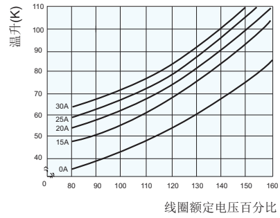
线圈温升
