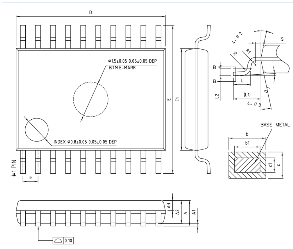
图 7-5 TSSOP20 封装尺寸图
