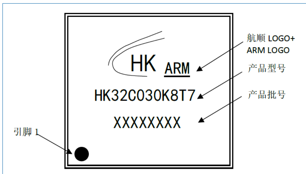
图 7-8 LQFP32 丝印示例 (HK32C030K8T7)
