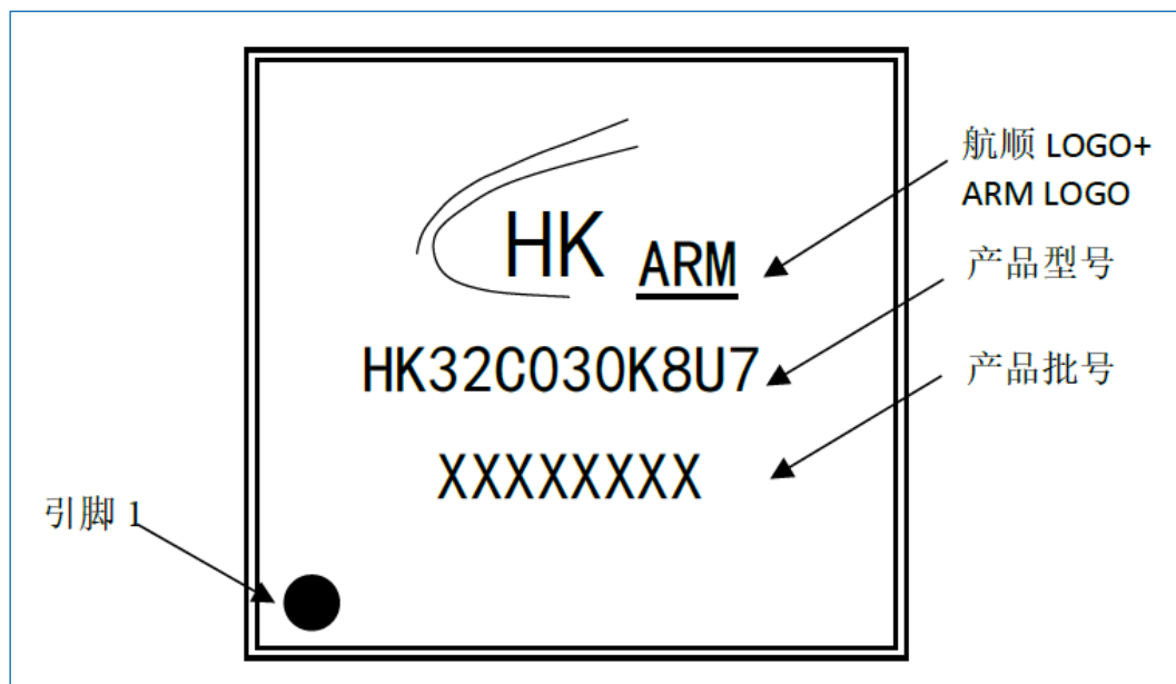
图 7-9 QFN32 丝印示例 (HK32C030K8U7)
