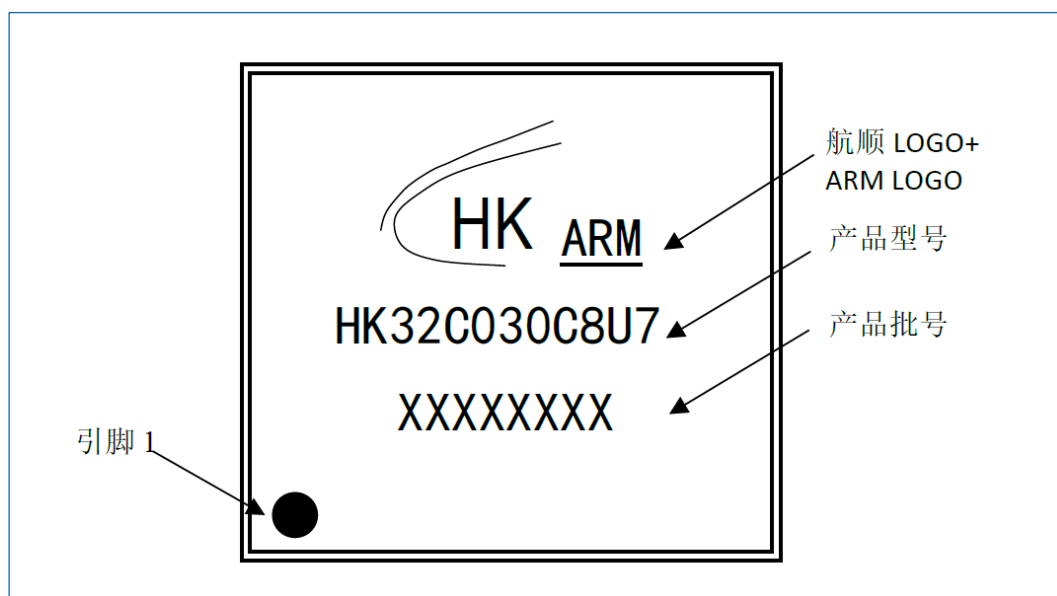
图 7-6 QFN48 丝印示例 (HK32C030C8U7)
