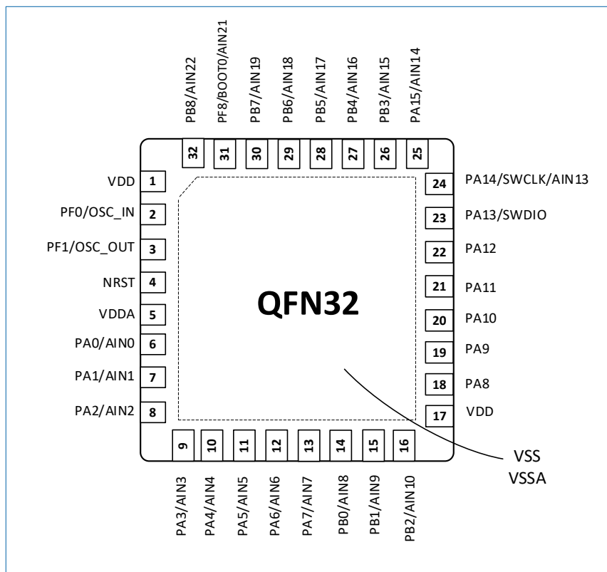
图 6-4 QFN32 封装引脚排列
