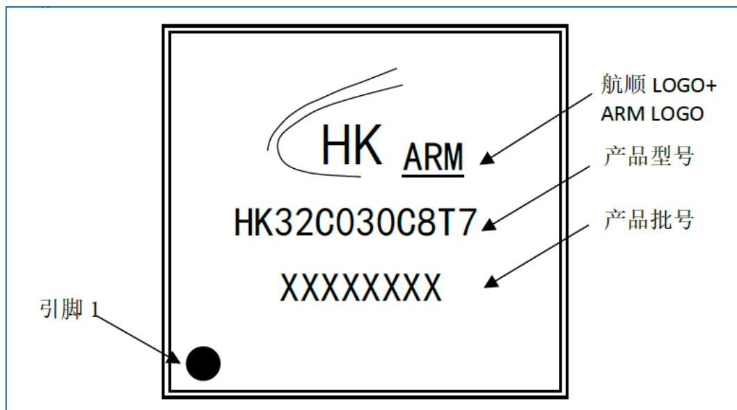
图 7-7 LQFP48 丝印示例 (HK32C030C8T7)
