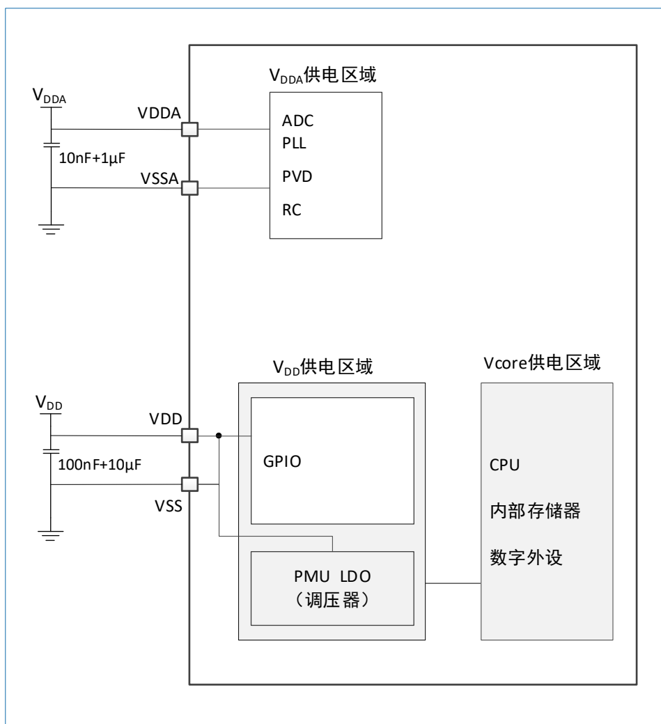
图 5-1 电源框图
