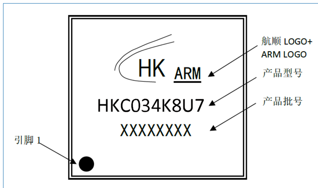
图 7-10 QFN32 丝印示例 (HK32C034K8U7)
