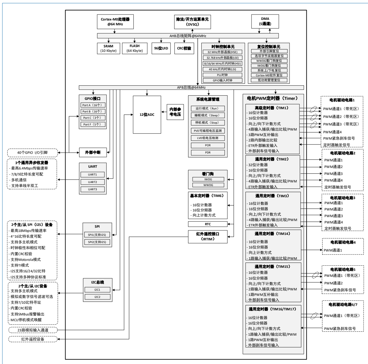
图 3-1 HK32C030C8T7 功能框图
