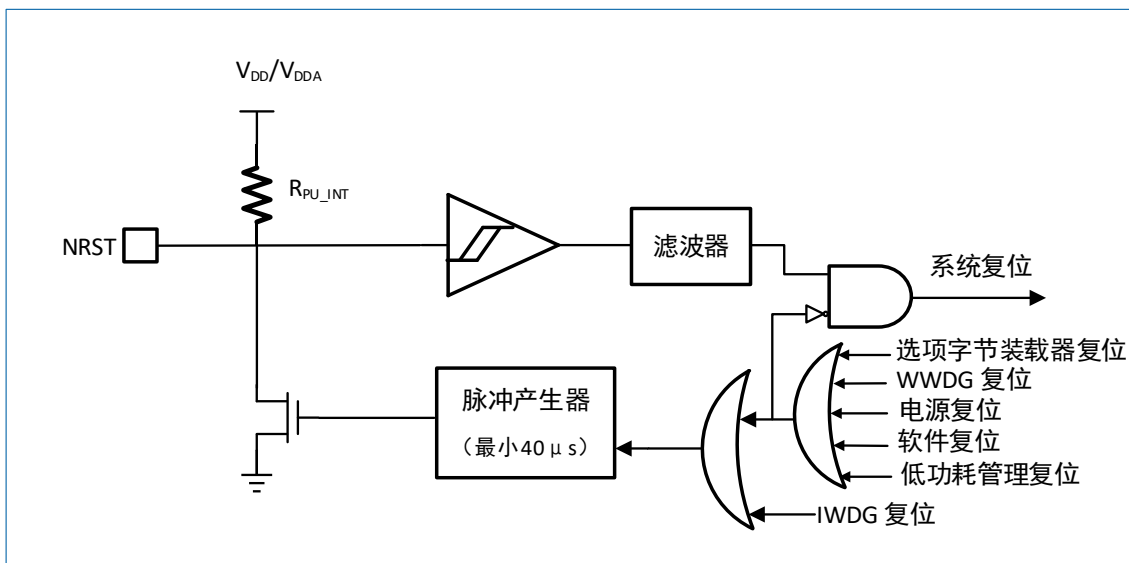
图 3-3 复位信号
