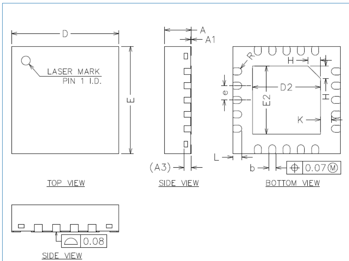
图 7-4 QFN20 封装尺寸 1
