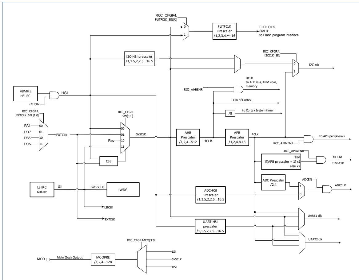
图 3-4 HK32F0301MxxxxC 时钟树
