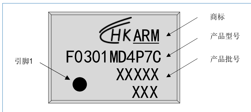
图 7-7 TSSOP16 HK32F0301MD4P7C 丝印示例
