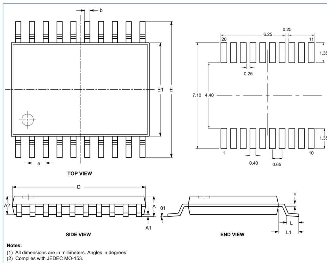
图 7-3 TSSOP20 封装尺寸
