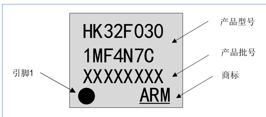
图 7-9 QFN20 HK32F0301MF4N7C 丝印示例
