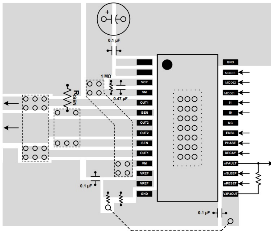
图 9. SS6952A 布局实例
