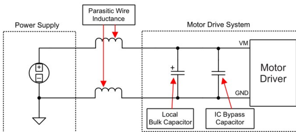
图 8. 外置电源电机驱动系统的设置
