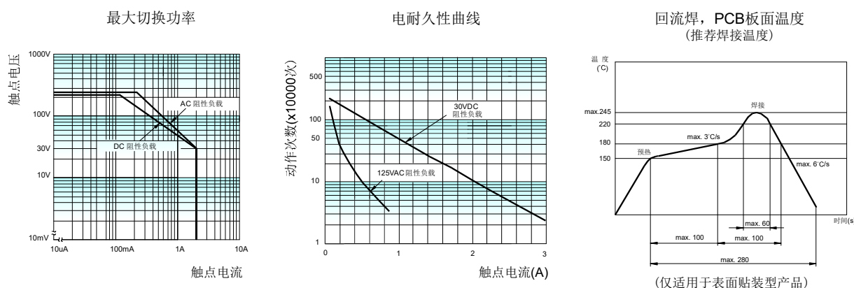
性能曲线图
