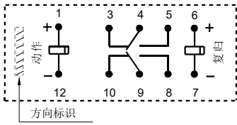
图示为复归状态
