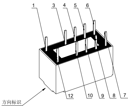
双线圈磁保持
