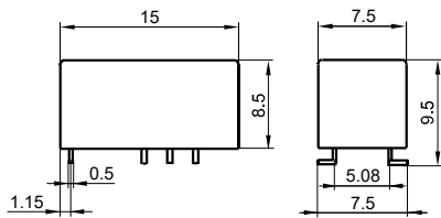
双线圈磁保持
