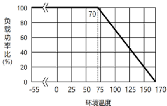
功率曲线
