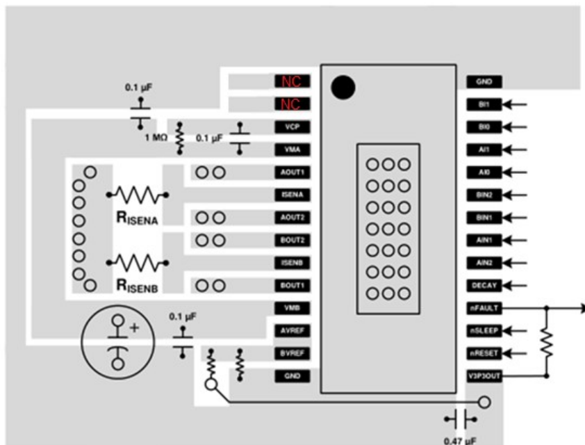
图 9. SS8841T 布局实例
