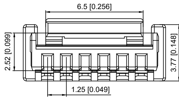
SEC:A-A
