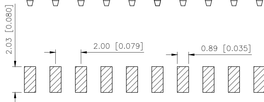
P.C.B LAYOUT
