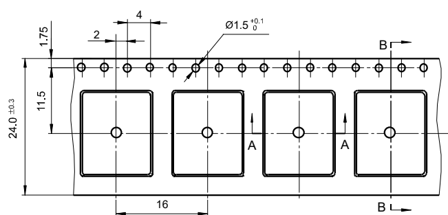
载带外形图 (S型: 标准表面贴装型)
