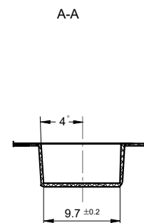
载带外形图 (S1型: 短脚表面贴装型)
