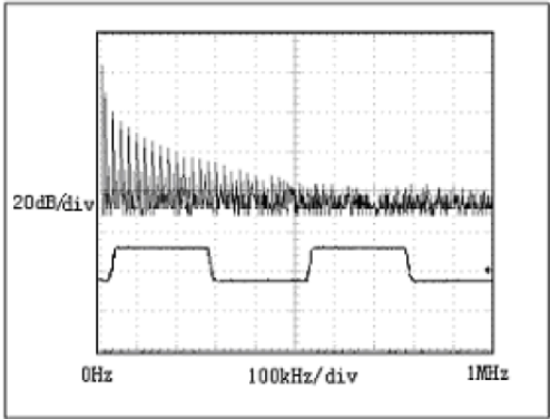
图11：传输20kHz信号时 MAX3485ESA+TD驱动器输出波形和FFT图
