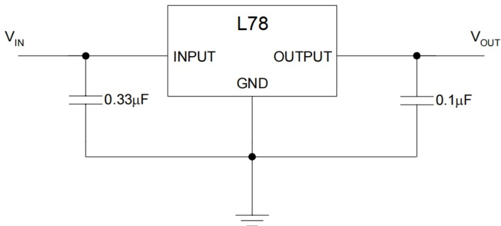
图 1. 典型应用原理图
