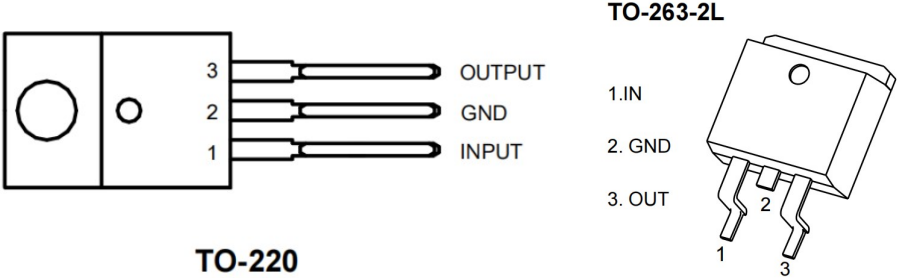
图 2. 引脚图
