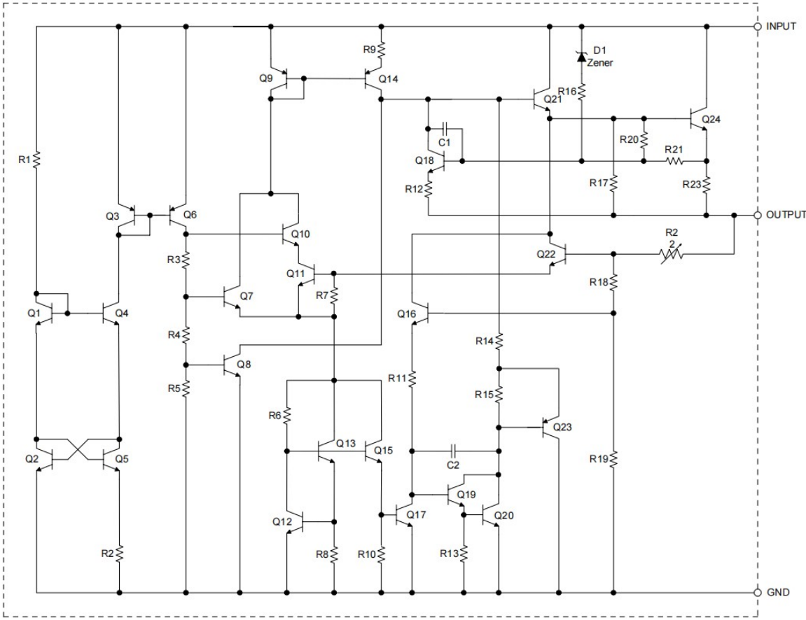
图 3. 功能框图
