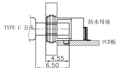
组装示意图
