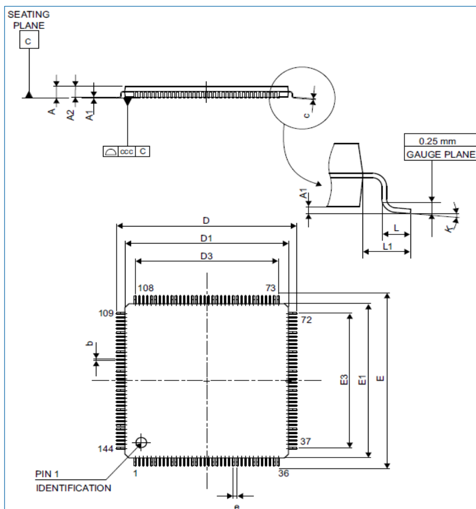
图 7-4 LQFP144 封装尺寸
