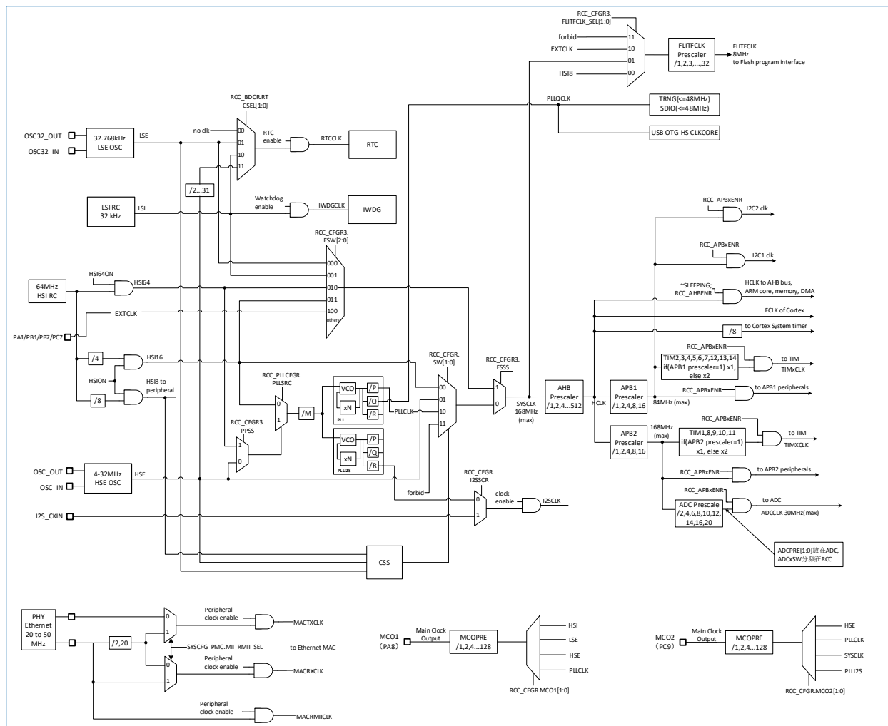
图 3-4 时钟树
