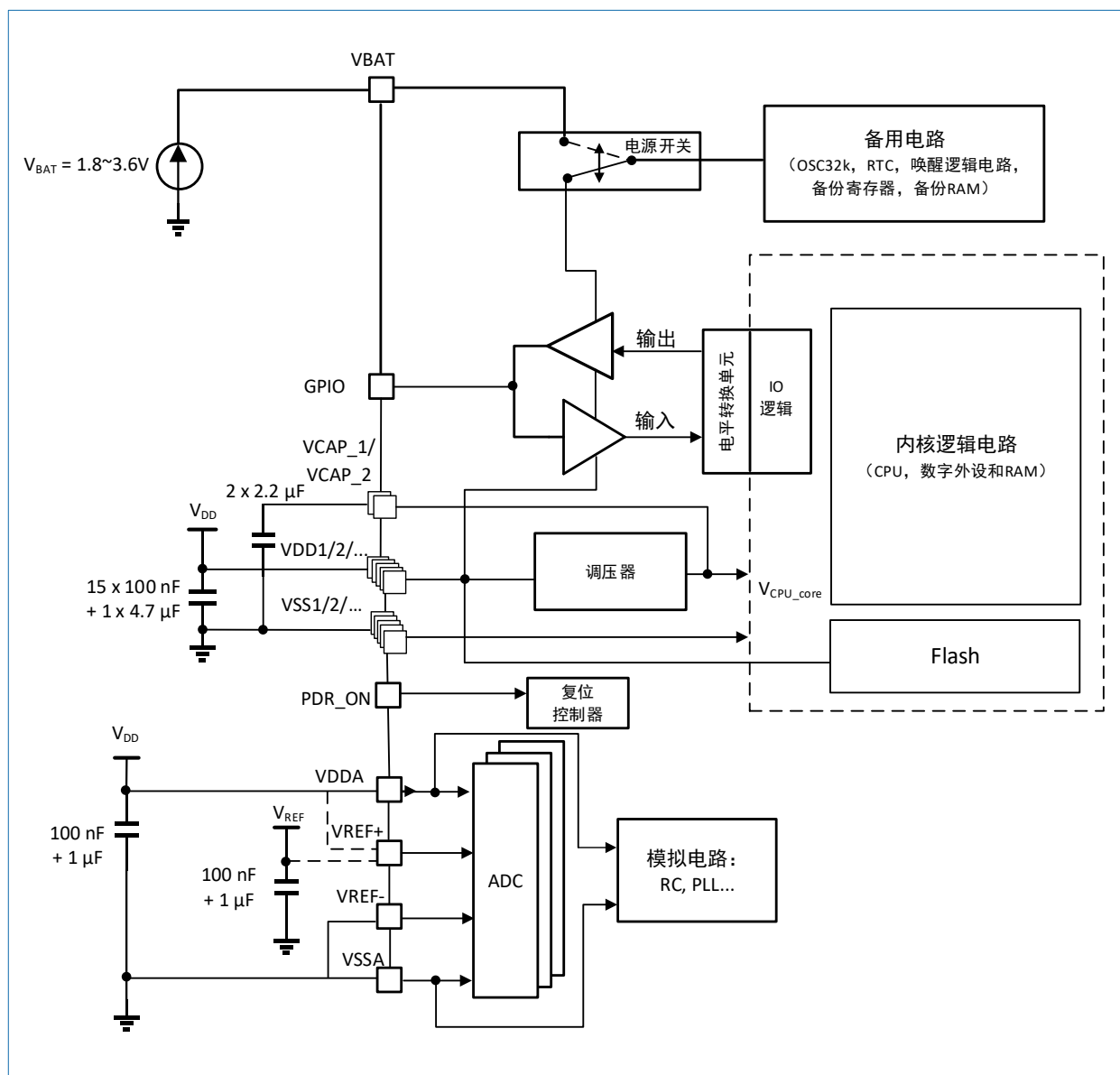
图 5-1 电源供电
