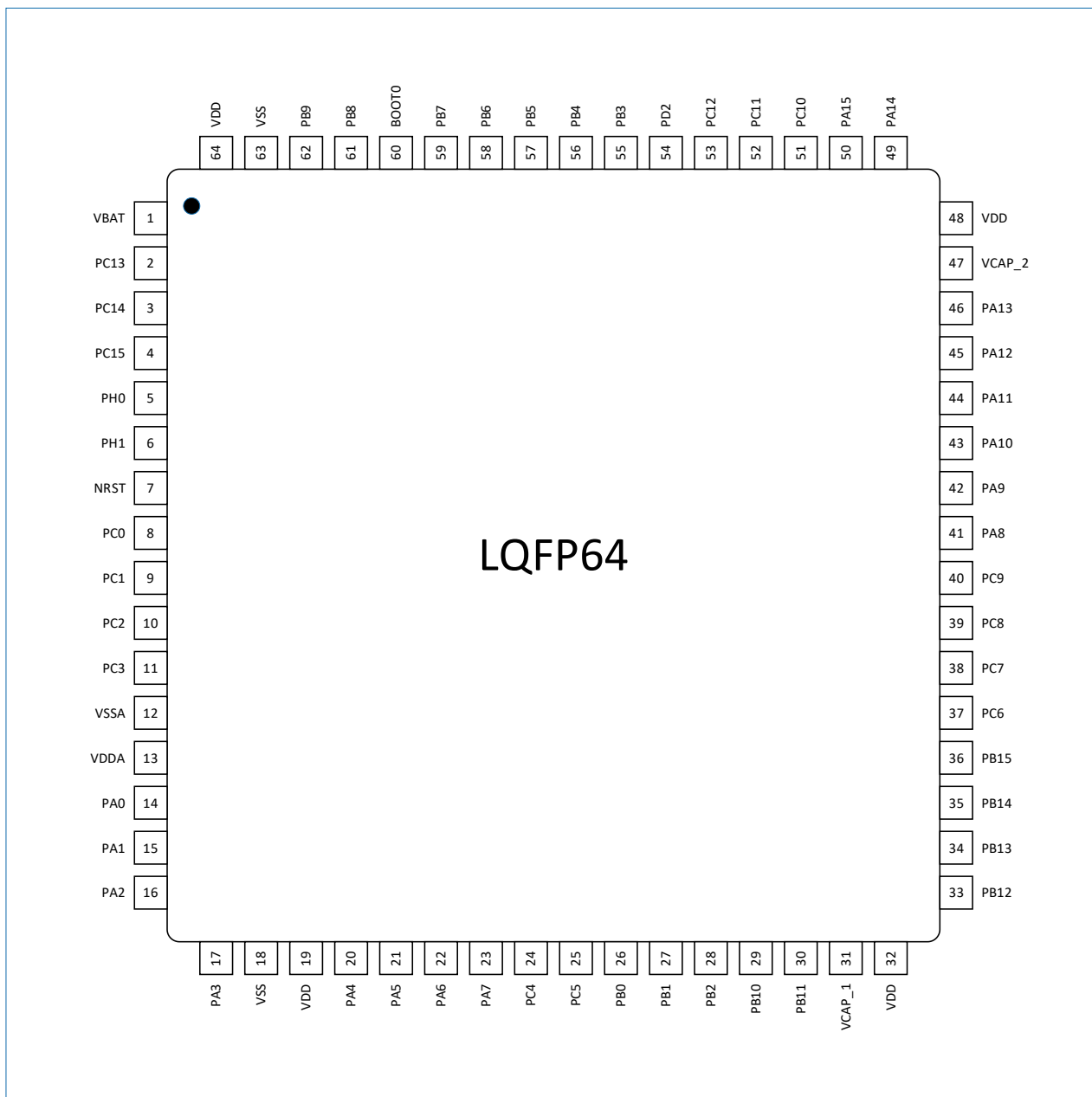
图 6-2 LQFP64 封装
