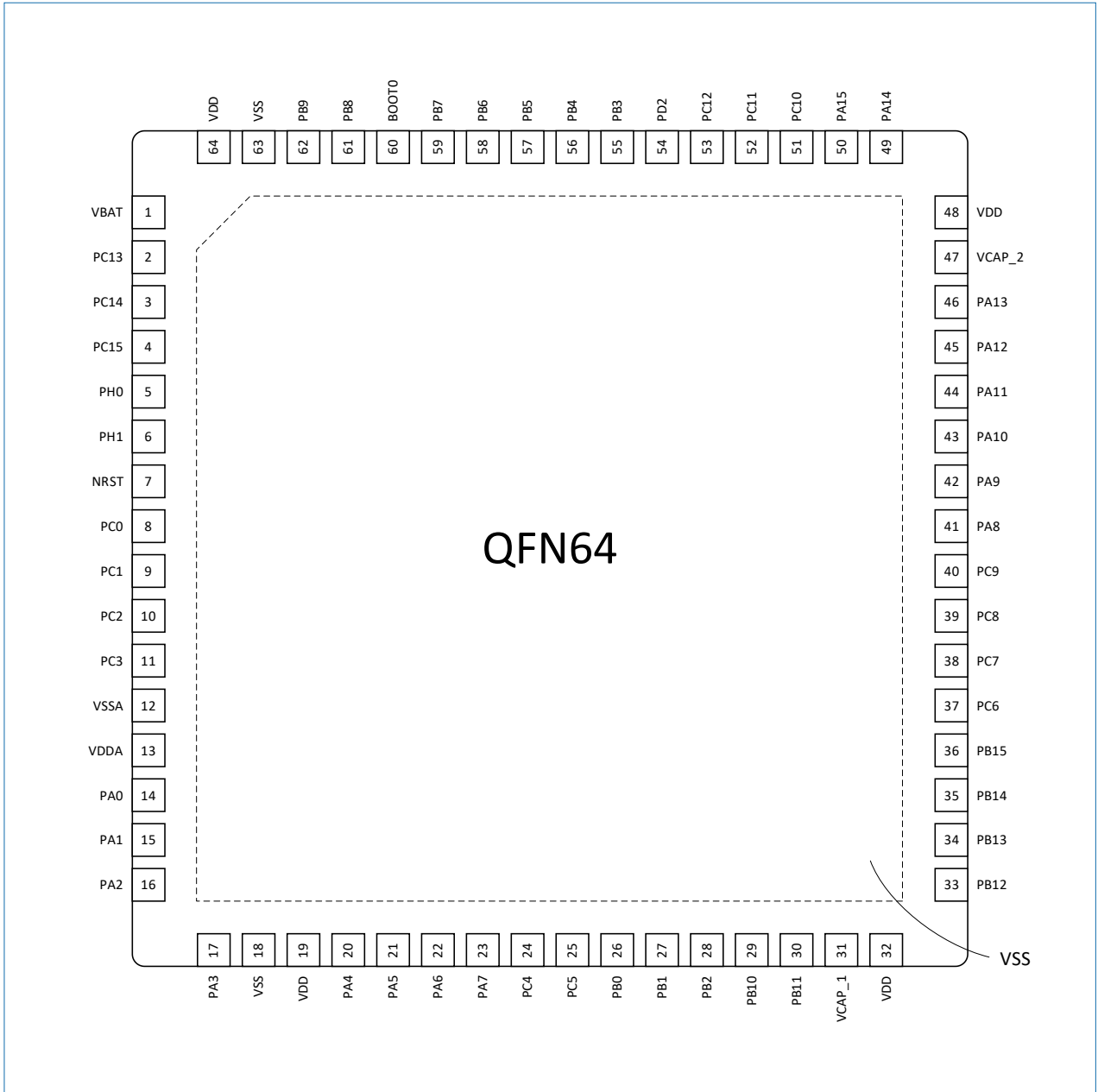
图 6-1 QFN64 封装
