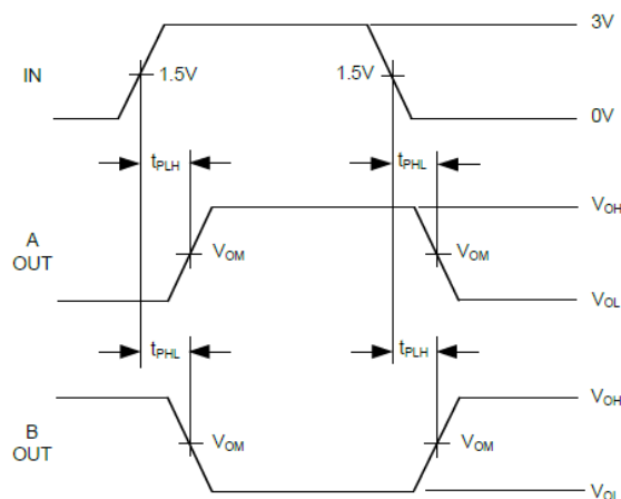
图 2 接收 V_{OH} 和 V_{OL}
