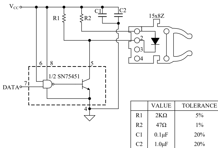
图 3 NRS15x8Z 典型应用电路图
