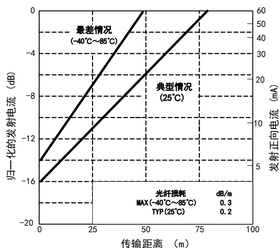
图1 配合 1mm 芯径 POF 光纤 NRS15x8Z/25x8Z 传输距离极限
