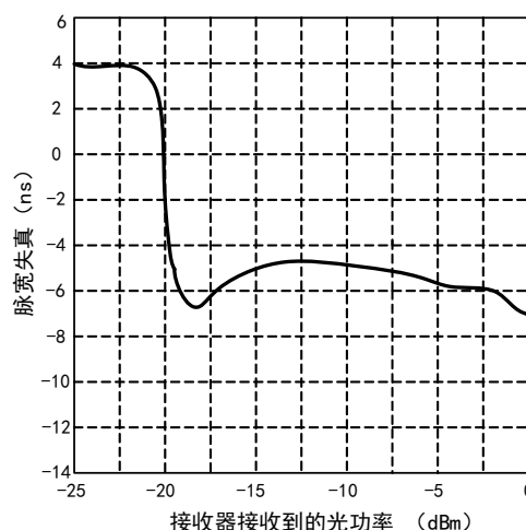
图2 在 10MBd 速率下 NRS15x8Z/25x8Z 的脉宽失真
