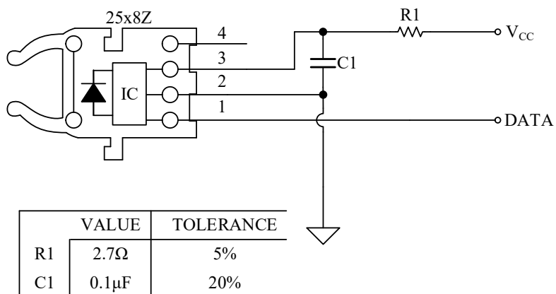
图 4 NRS25x8Z 典型应用电路图
