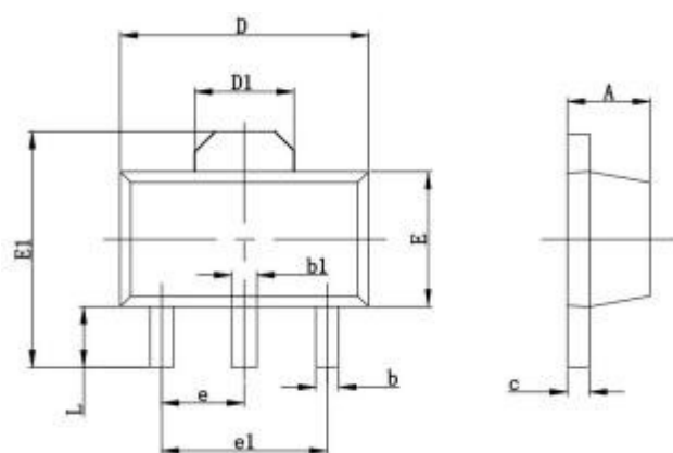
SOT-89-3L
