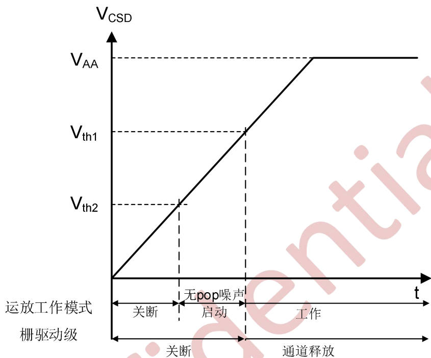
图 10-5 NSA2092 V_{CSD} 和运算放大器的工作模式
