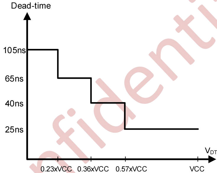
图 10-6 NSA2092 中死区时间与 V_{DT} 的关系
