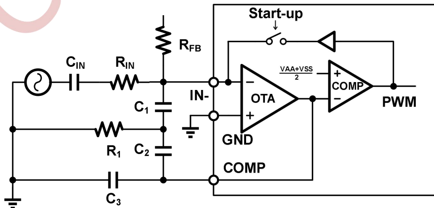
图 10-4 NSA2092 “咔哒”噪声消除机制
