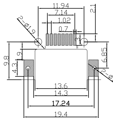
PCB参考图
