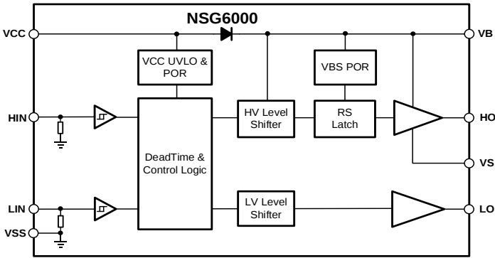
简化示意图
