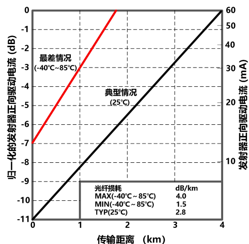
图 8 配合 62.5/125μm 芯径光纤 NRS1414xx/HFBR-2412 传输距离极限
