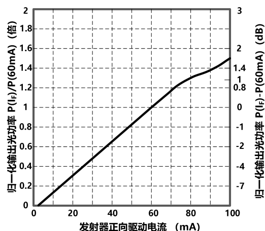
图 4 正向驱动电流与归一化输出光功率曲线
