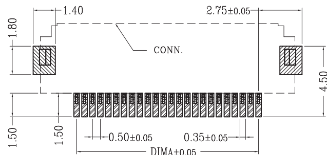
适用线路板 (PCB LAYOUT)
