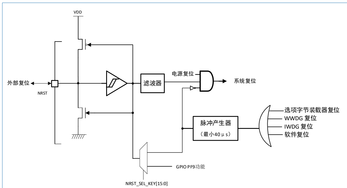
图 3-3 复位信号
