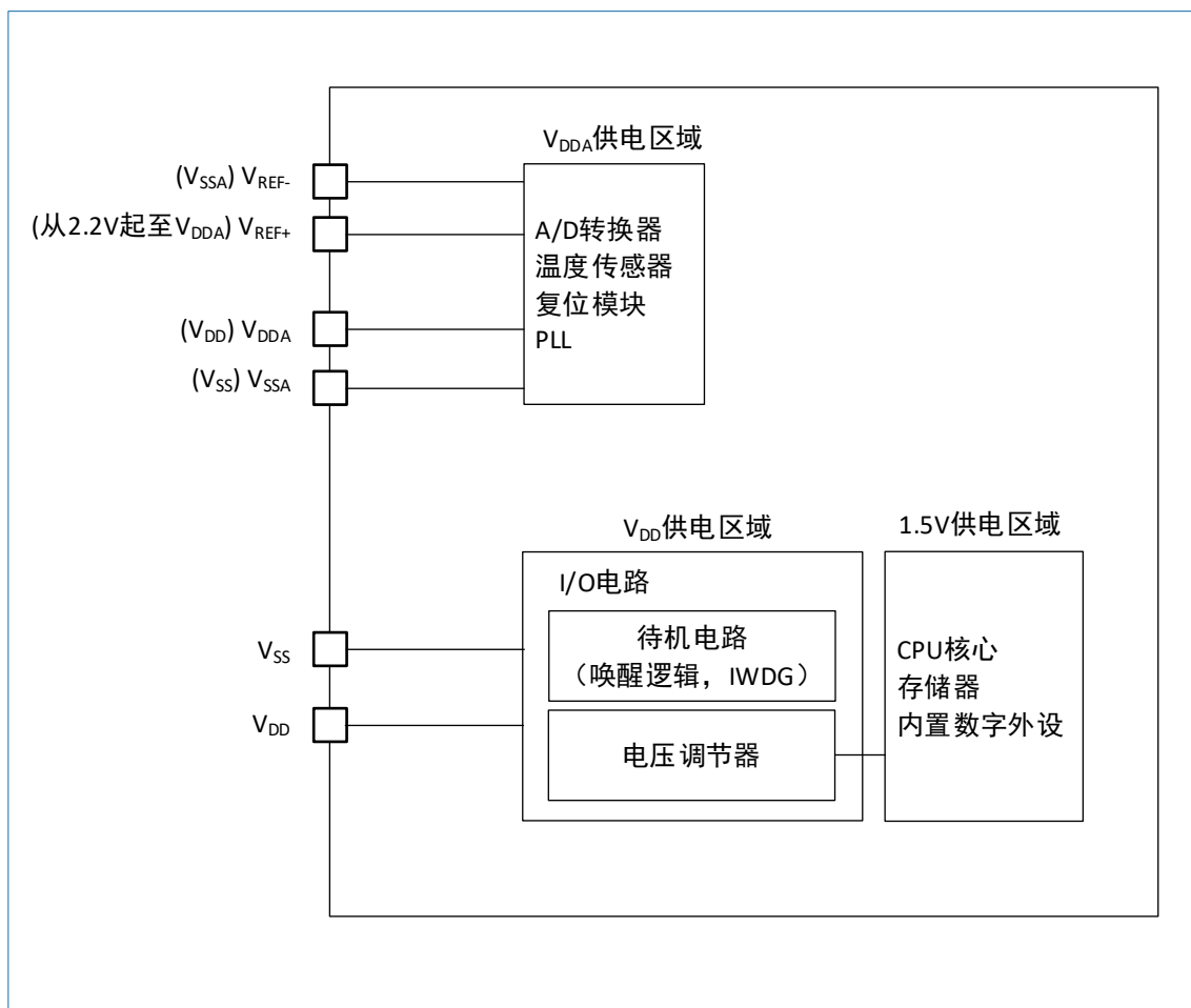
图 5-1 电源框图
