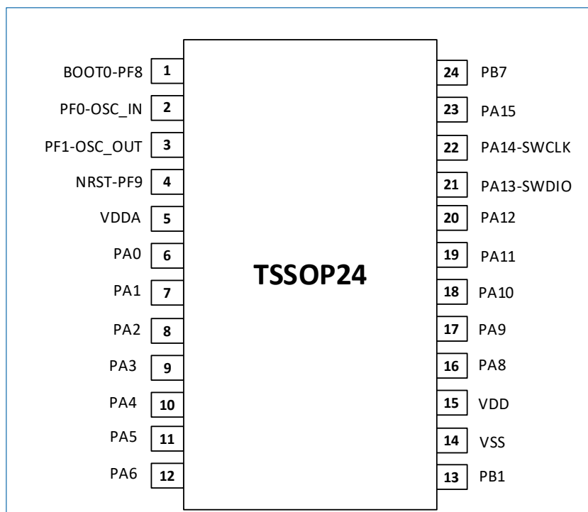
图 6-5 TSSOP24 封装引脚排列
