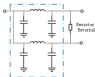
原理框图
