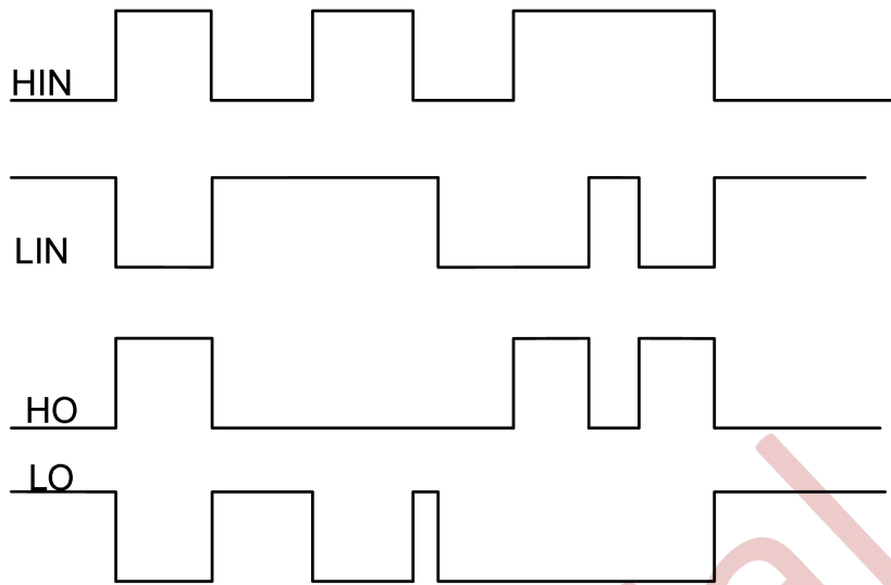
图 9-1 XJNG2102 输入输出时序波形
