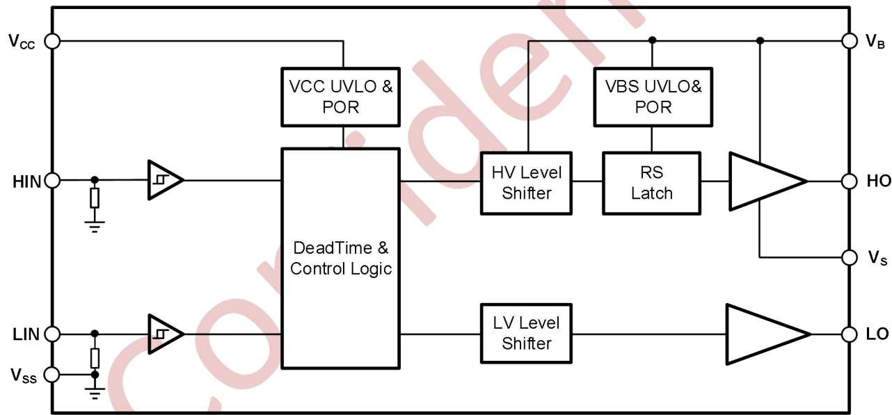
图 10-1 XJNG2102 功能框图
